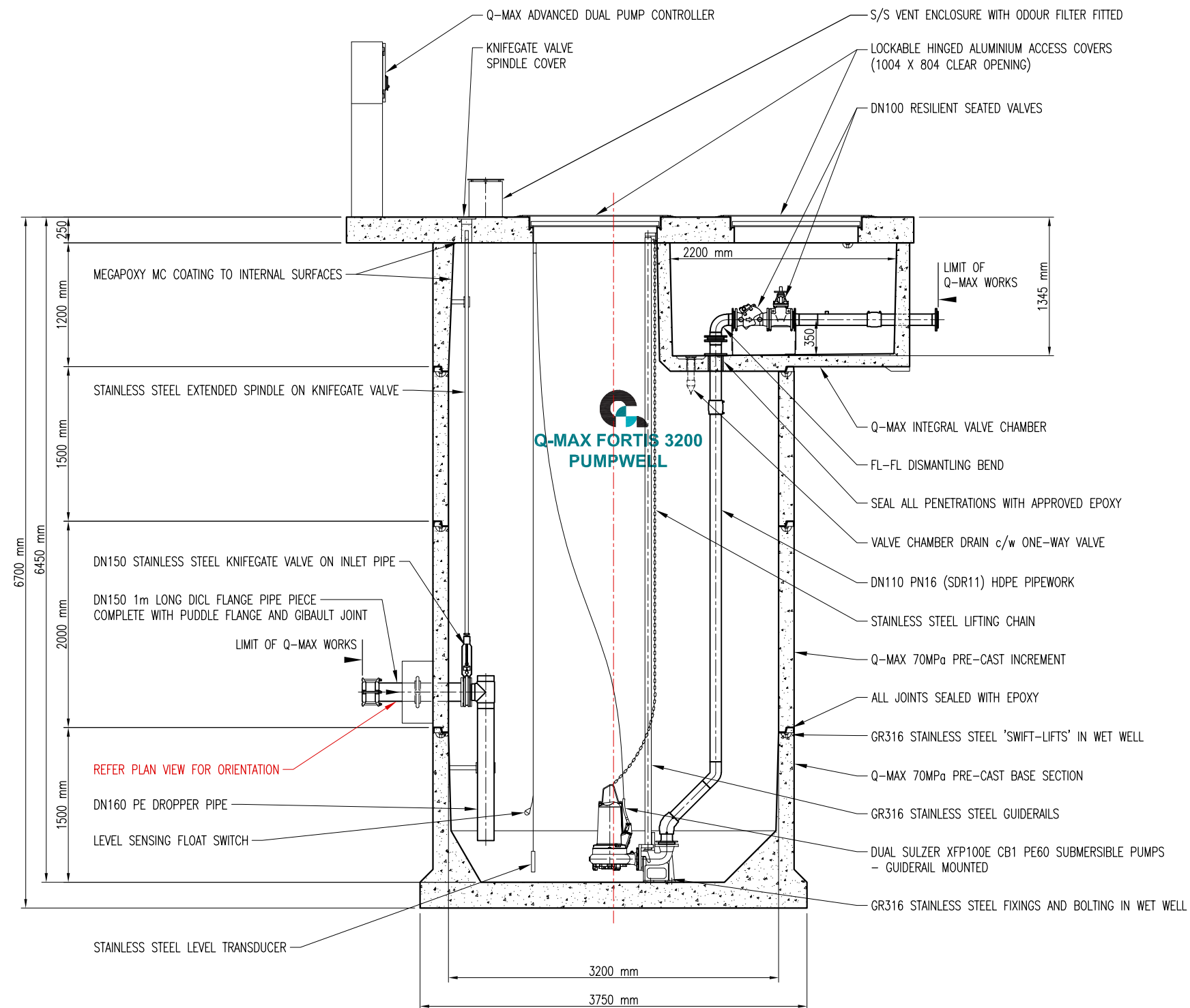
SECTIONAL ELEVATION SCALE: 1 : 50 @ A3
